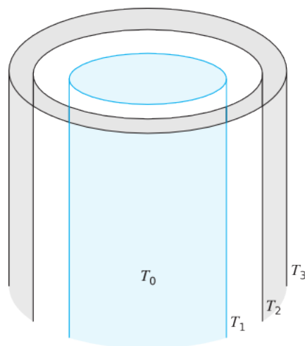
Figura 1: Envase térmico.
